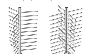
90°/ 120° Rotor (drei oder vier Abschnitte)
